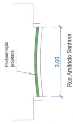
3 Seção Transversal Escala: 1:25
