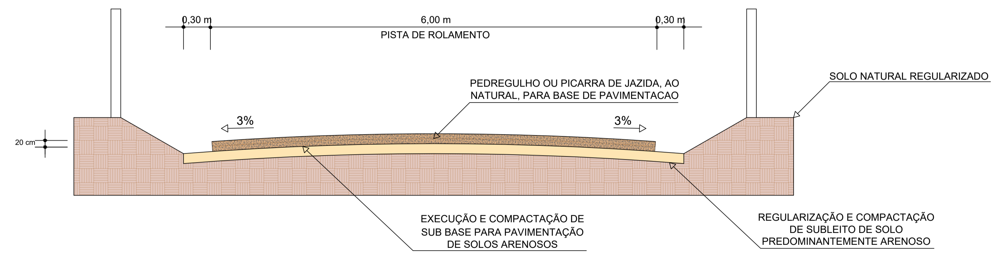
SEÇÃO TRANSVERSAL TIPO
