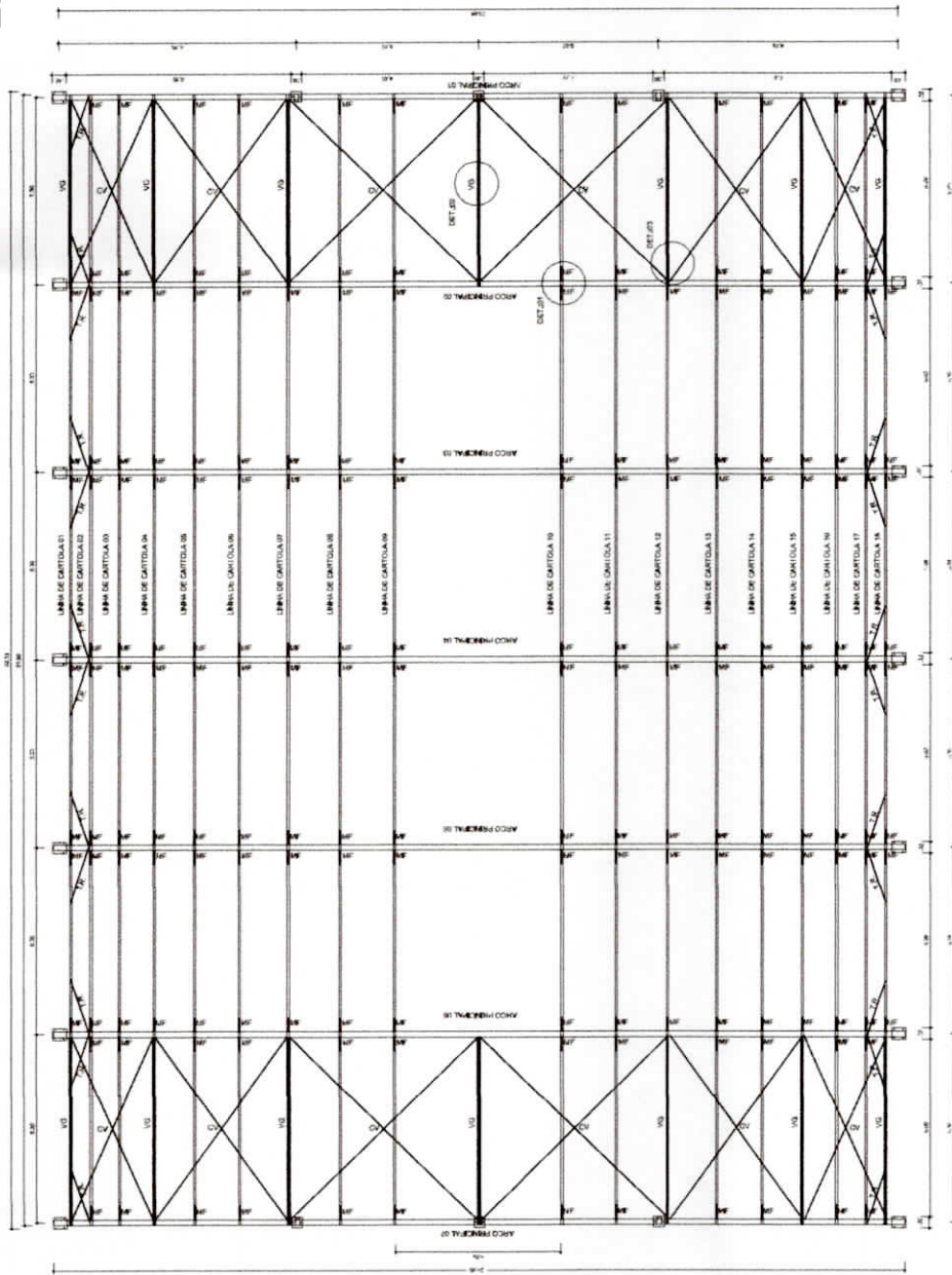
PLANTA BACIA ESCALA: 1/75
