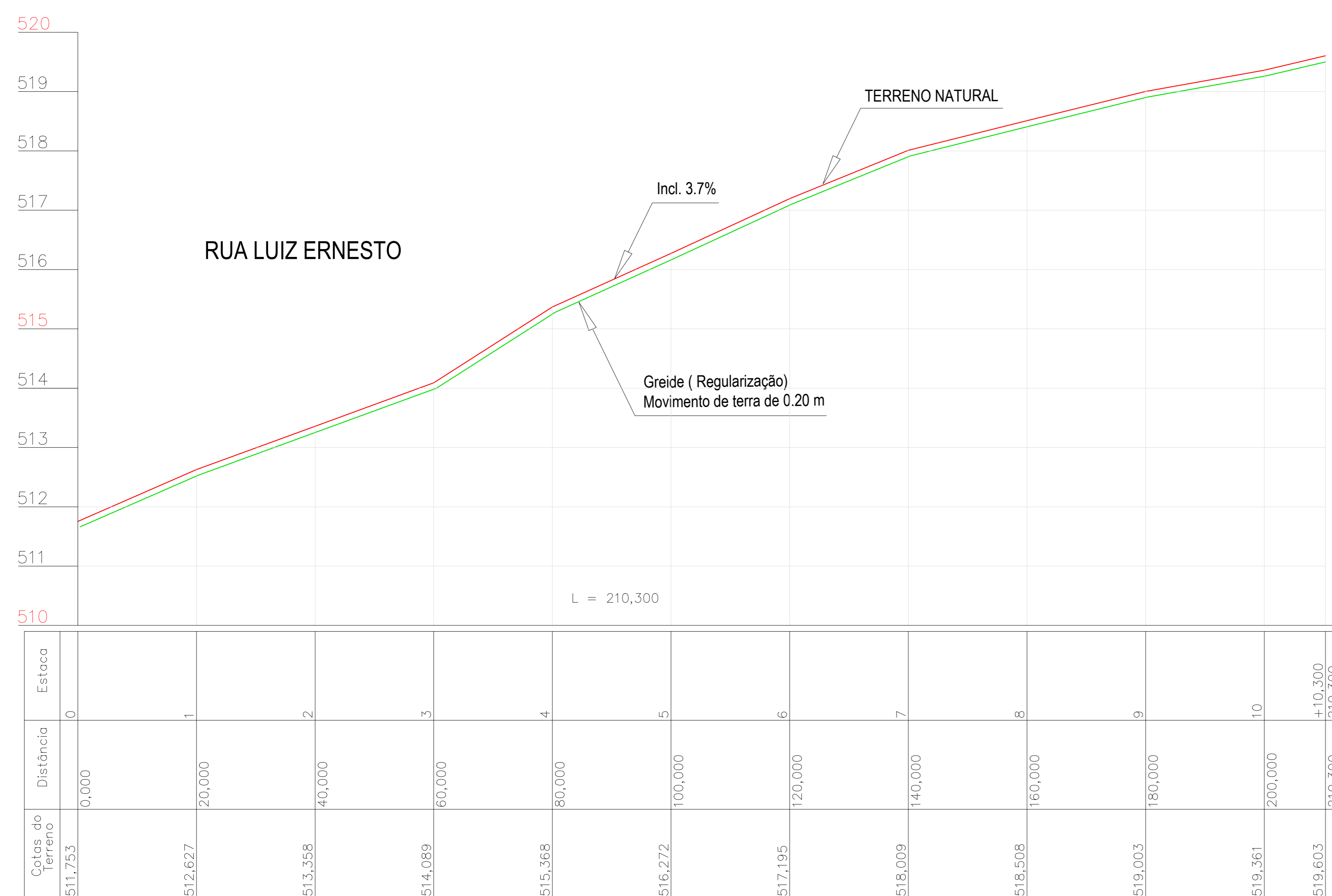
PERFIL LONGITUDINAL Esc. Horizontal: 1/500 Vertical: 1/50
