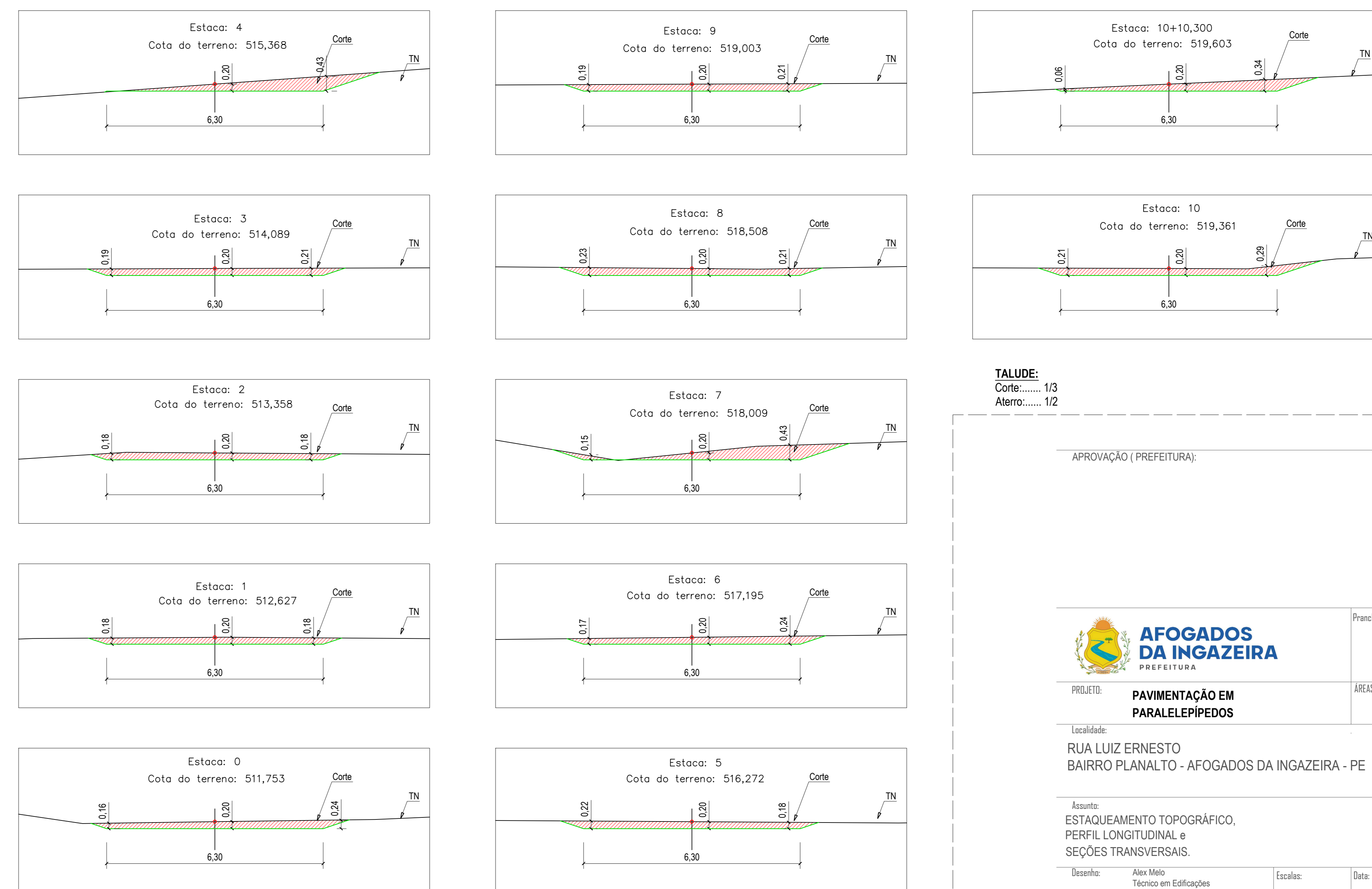
SEÇÕES TRANSVERSAIS ( Rua Luiz Ernesto ) Esc. 1/75
