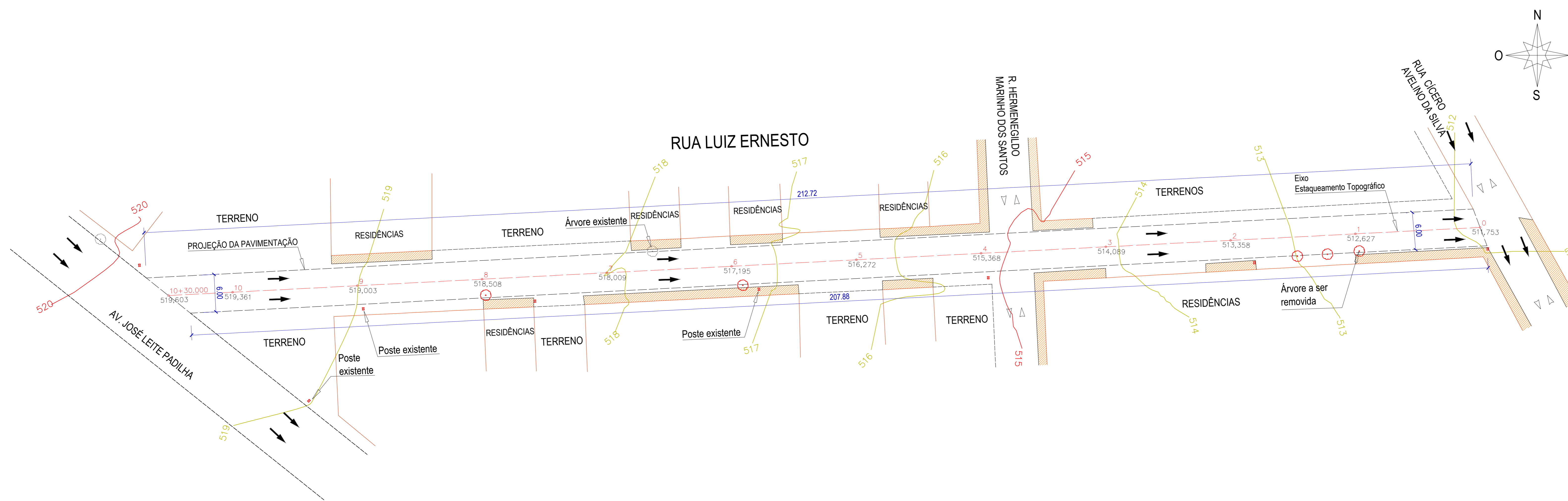
ESTAQUEAMENTO TOPOGRÁFICO Esc. 1/300
