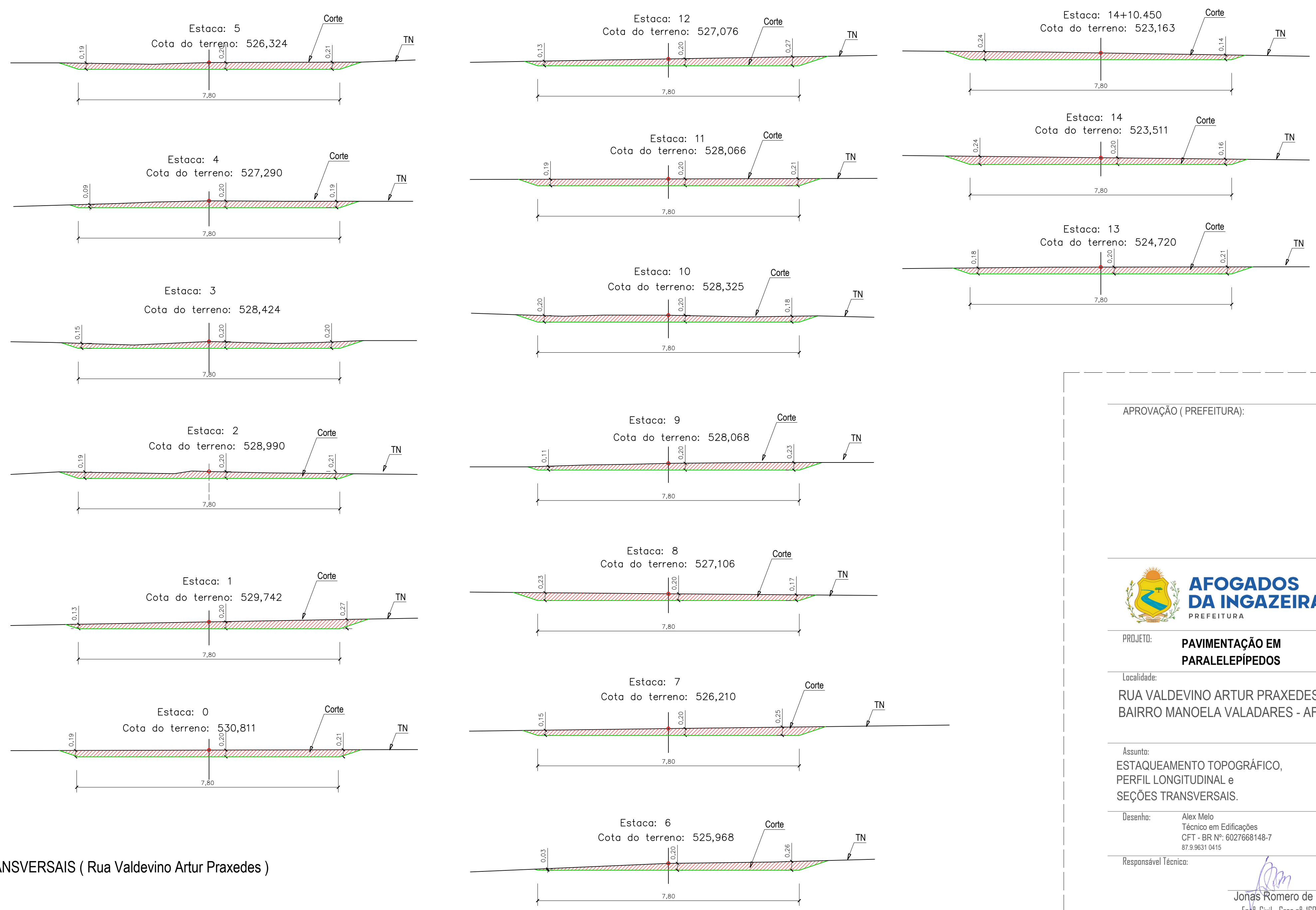
TALUDE: Corte:..... 1:3 Aterro:..... 1:2
