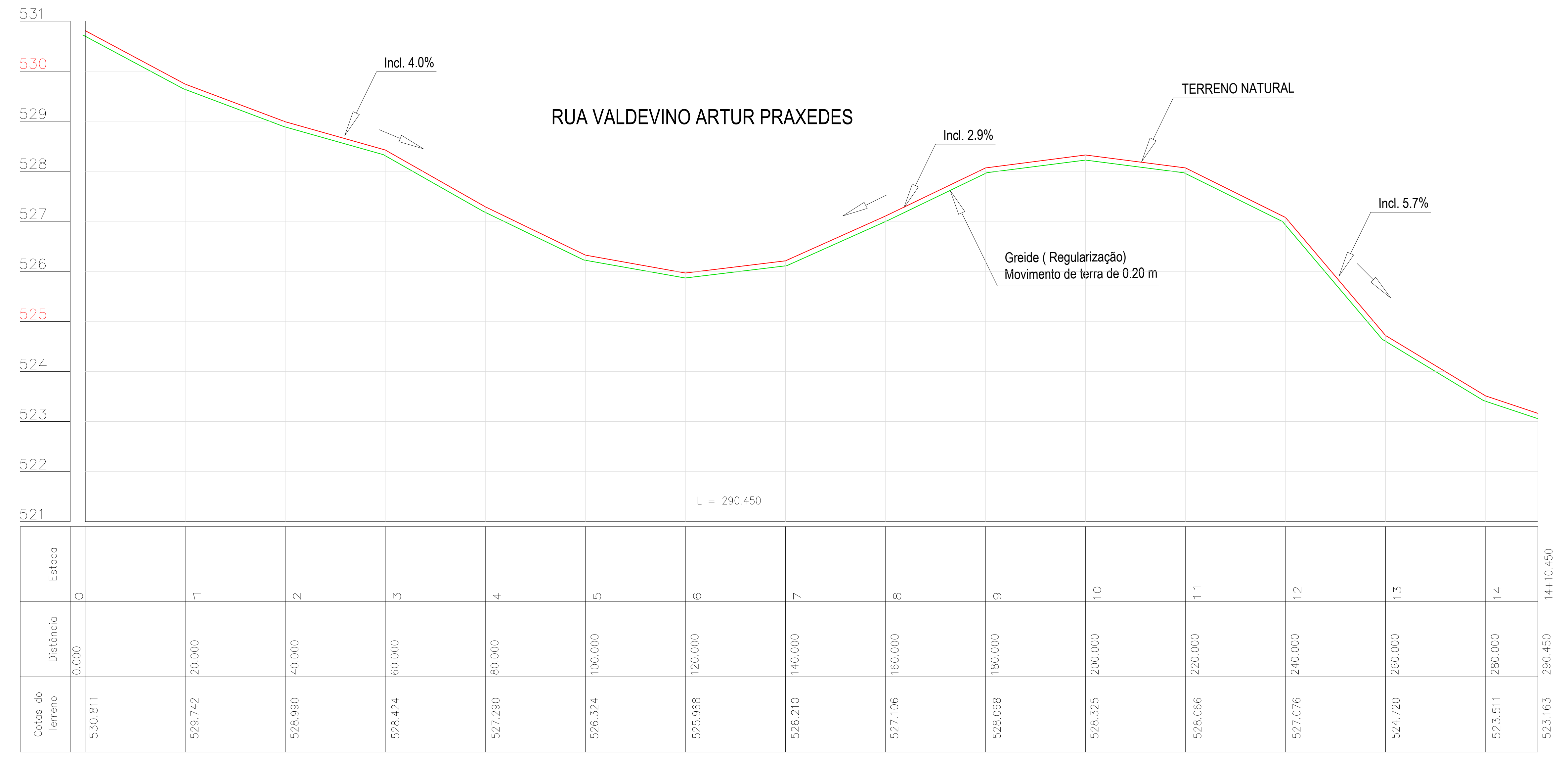
PERFIL LONGITUDINAL Esc. Horizontal: 1/500 Vertical: 1/50
