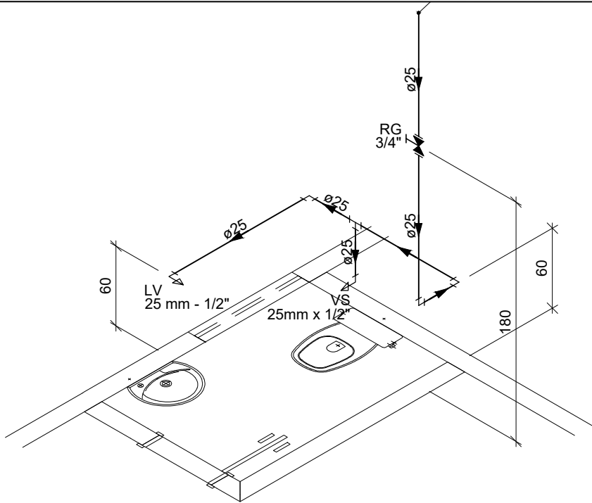
Detalhe H3 Escala 1:40
