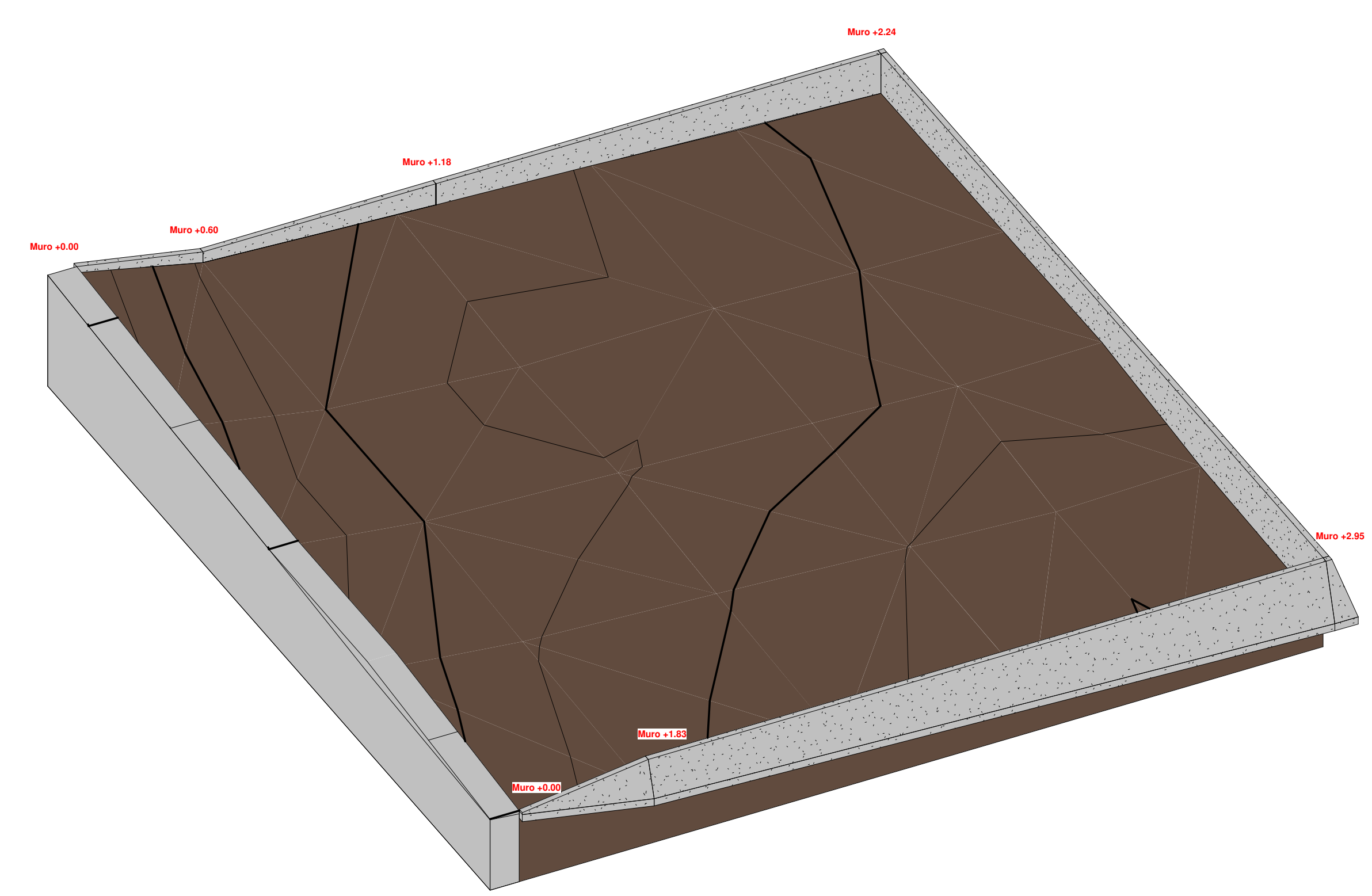
3 3D - Solo do Aterro e Muro
