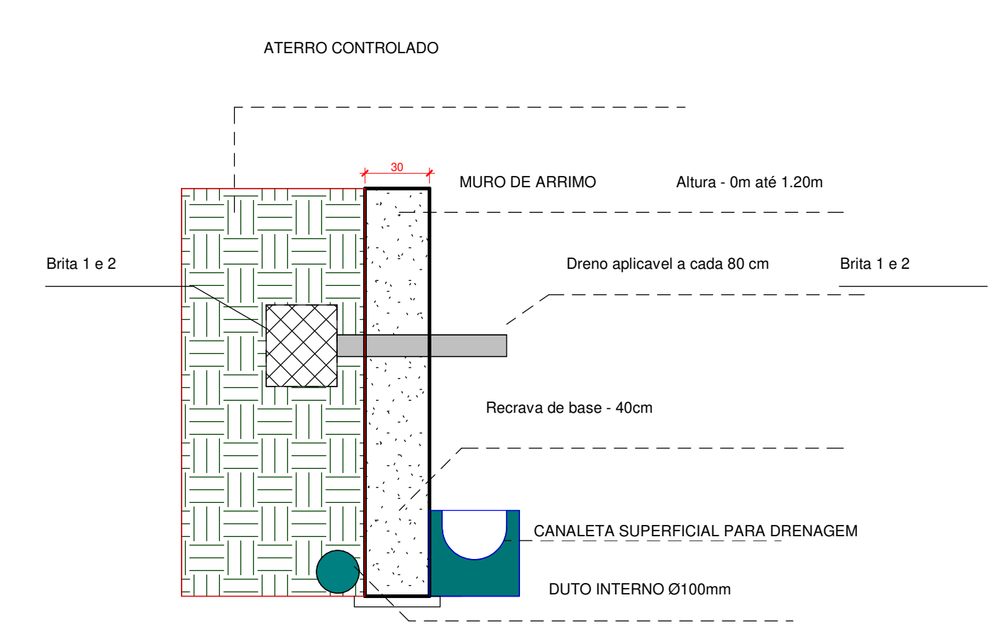
4 DETALHAMENTO DOS MUROS DE ARRIMO 1 : 25
