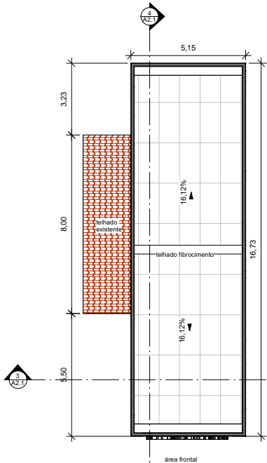
2 COBERTA 1 : 100
