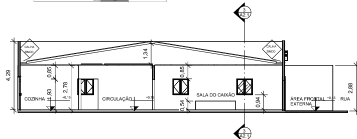
4 CORTE AB 1 : 100
