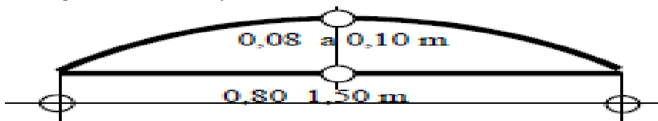
FIGURA – 2 – LOMBADA TIPO - 2
