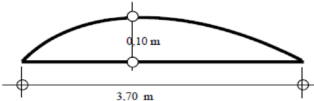
FIGURA – 2 – LOMBADA TIPO - 2
