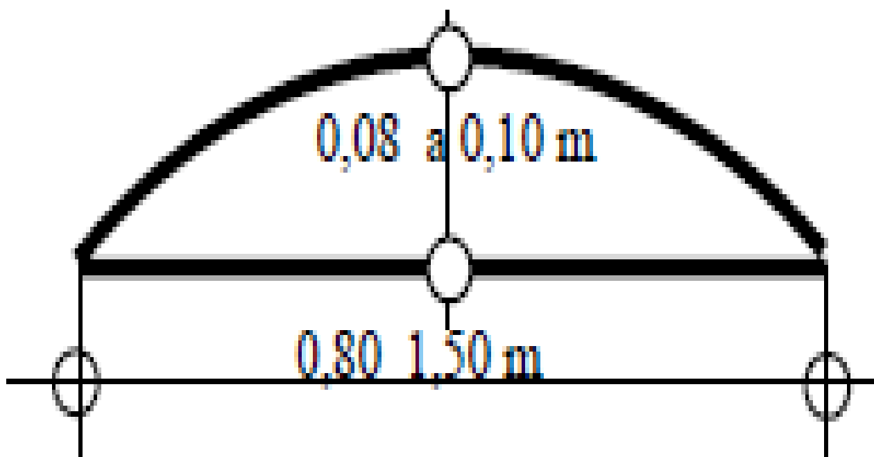
Figura 01- Lombada Tipo I
