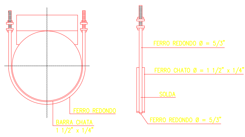
FLUTUANTE DETALHE 01 S/ESC.
