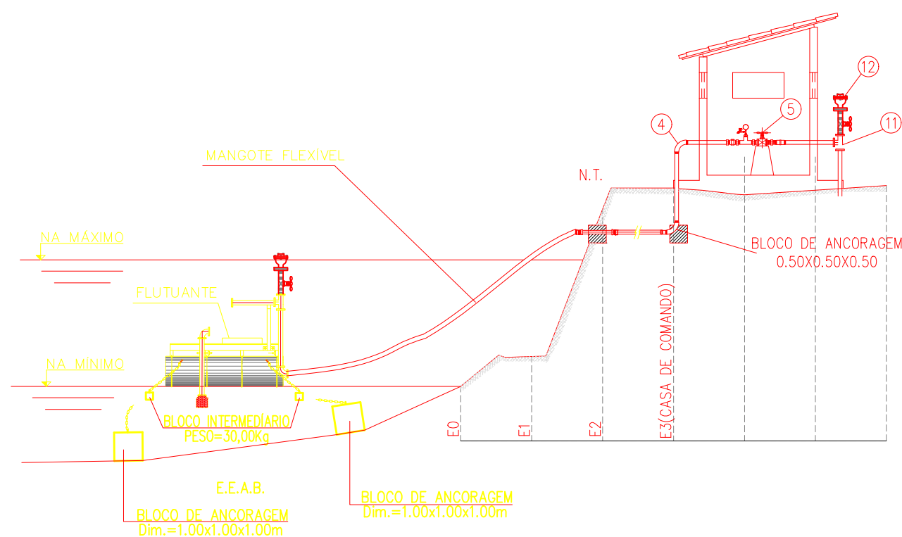
DETALHE DA CAPTAÇÃO SEM ESCALA
