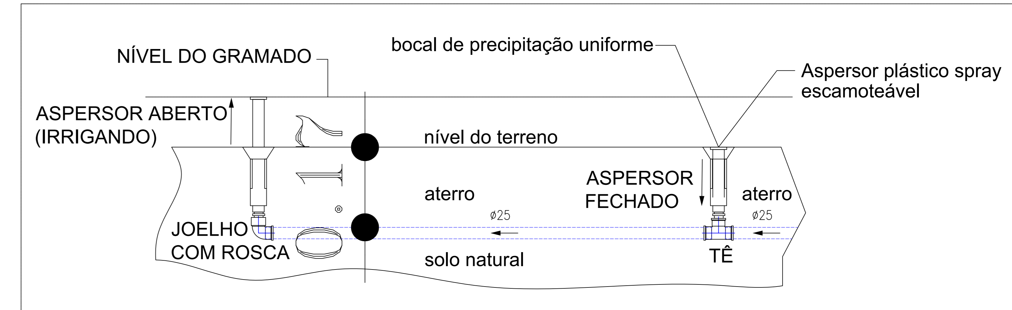
CORTE ESQUEMÁTICO DE MONTAGEM DOS ASPERORES APÓS OS JOELHOS DOS CANTEIROS ESCALA: 1/5
