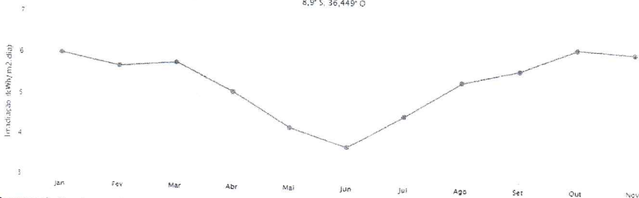
Irradiação Solar no Plano Inclinado -Garanhuns-Garanhuns, PE-BRASIL
