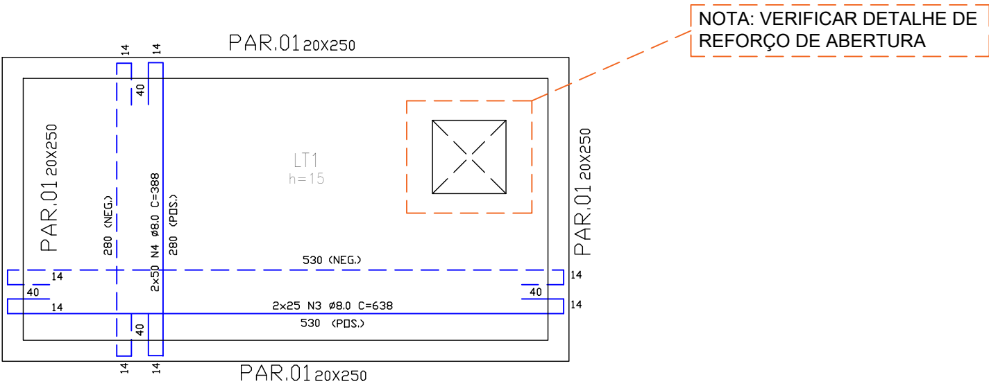
Det. amadura - laje de fundo Esc 1:50
