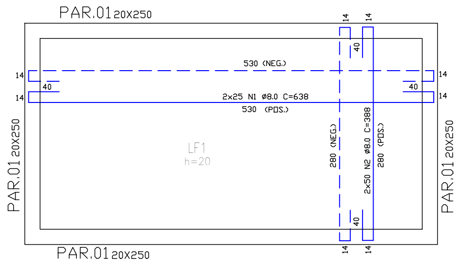
Det. amadura - laje de fundo Esc 1:50
