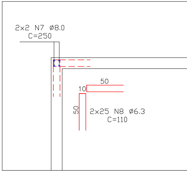
Detalhe arm. canto Esc 1:25
