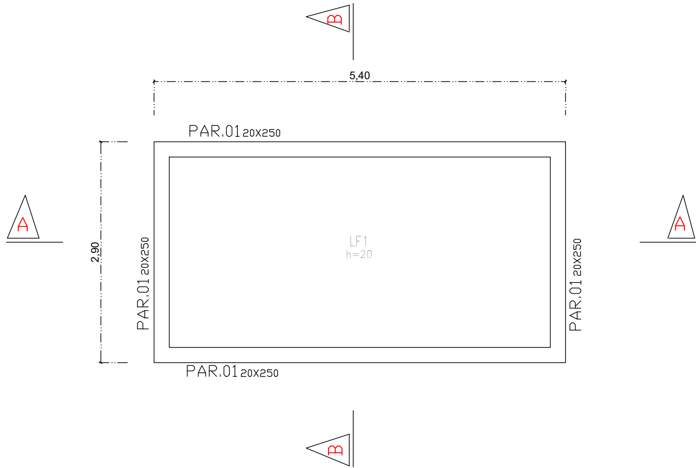
Planta Baixa - fundo (-2,5) Esc 1:50
