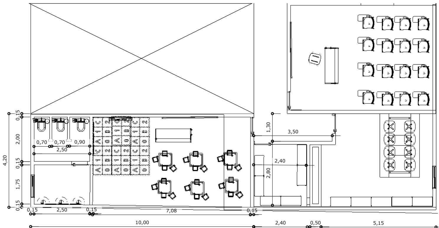
A4 1/100 Planta baixa - Alteração
